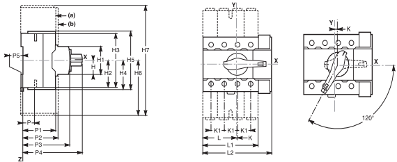
(a) Capa de proteção de terminal INS40/63/80. (b) Capa de proteção de terminal INS100/125/160.
