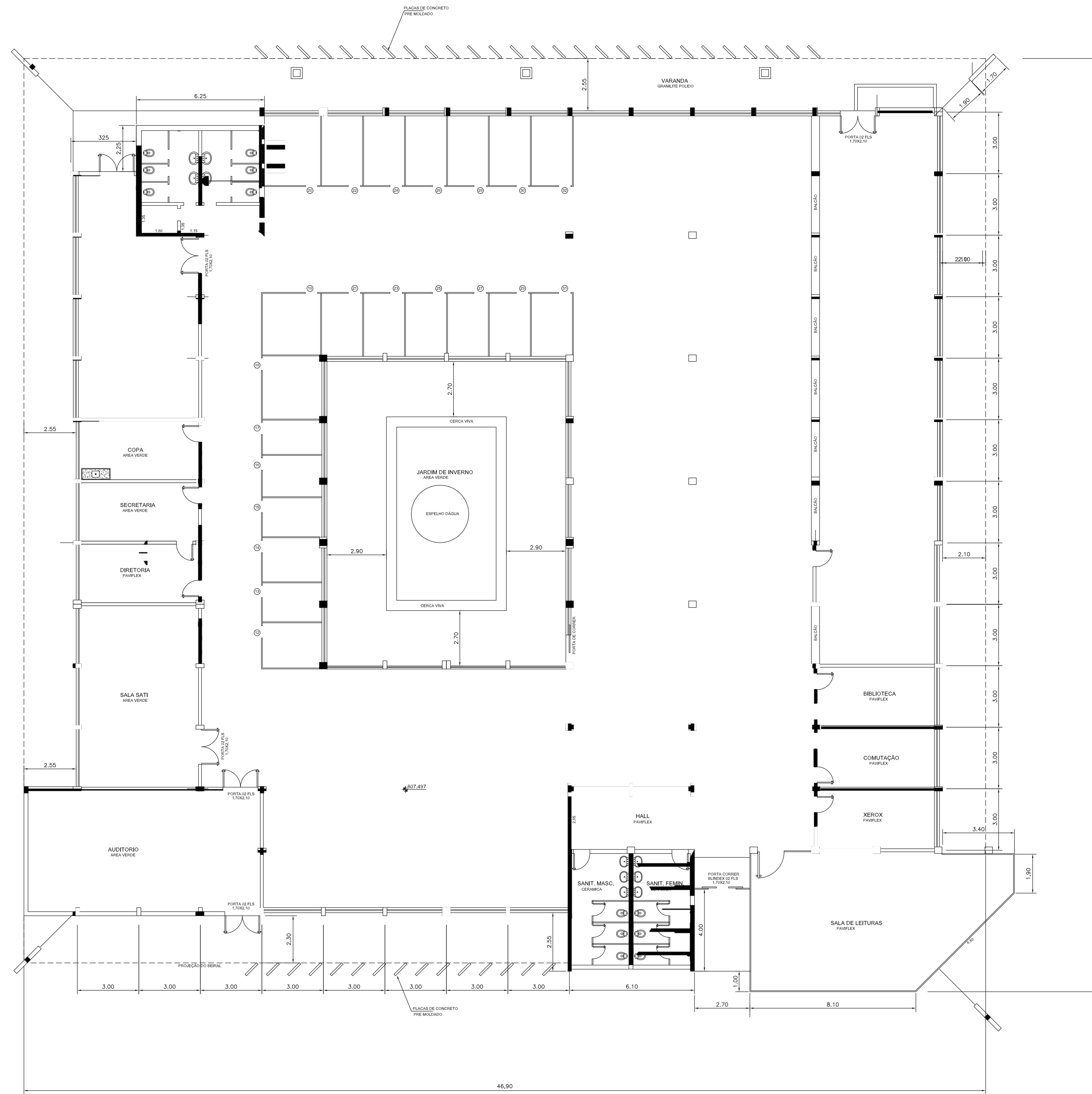
PLANTA DO PRÉDIO BIBLIOTECA ESCALA 1:100
