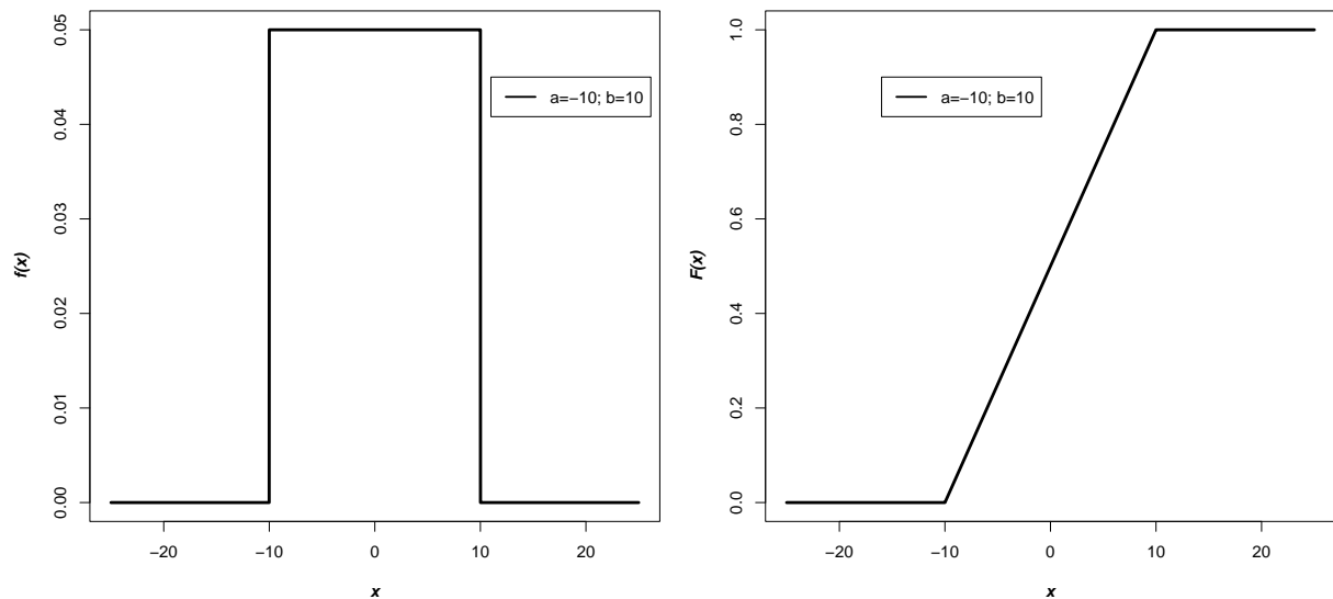
Figura 2.1: Distribuição uniforme
