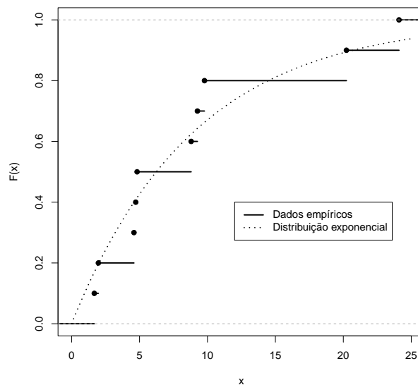
Figura 2.9: F_o(x_i) e F_e(x) para o teste de aderência de Kolmogorov-Smirnov
