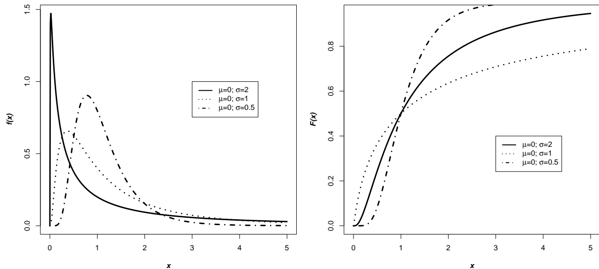
Figura 2.4: Distribuição lognormal
