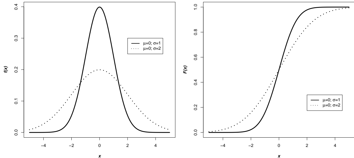
Figura 2.3: Distribuição Normal
