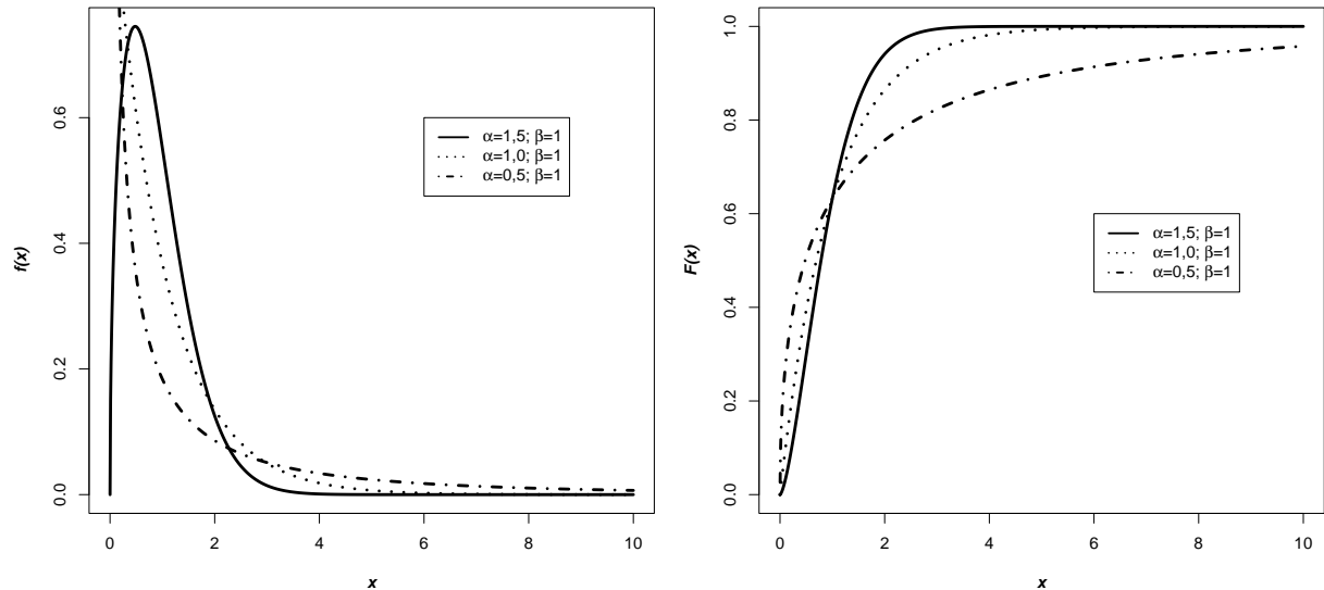
Figura 2.5: Distribuição de Weibull
