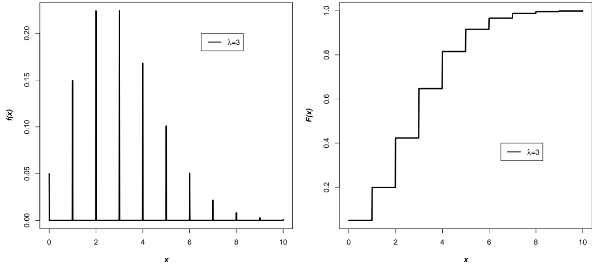
Figura 2.7: Distribuição de Poisson
