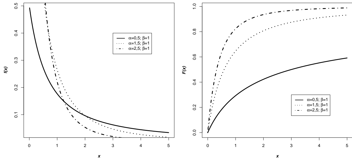
Figura 2.6: Distribuição de Pareto
