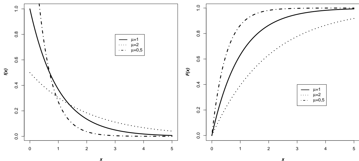
Figura 2.2: Distribuição Exponencial
